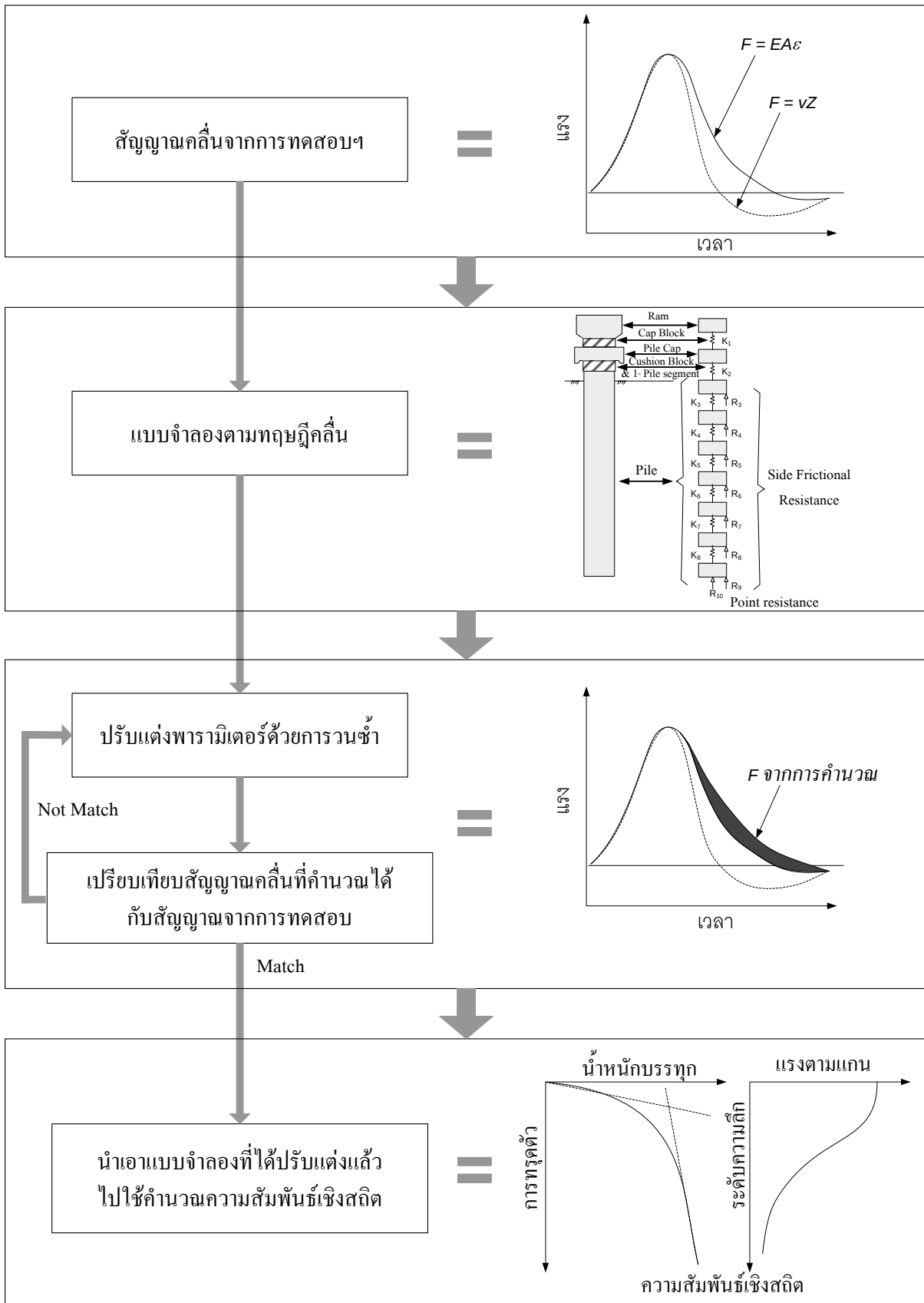
รูปที่ ค-4 ขั้นตอนการวิเคราะห์ด้วยกระบวนการงานจับคู่สัญญาณ
