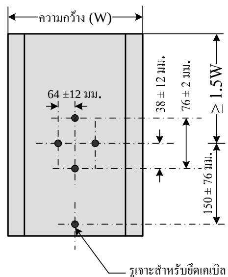
รูปที่ 6 ตำแหน่งแนะนำสำหรับการติดตั้งหัววัด สัญญาณเข้ากับเสาเข็มเหล็กรูปพรรณ (ข้อ 4.2)
