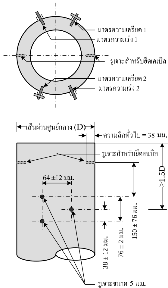
รูปที่ 4 ตำแหน่งแนะนำสำหรับการติดตั้งหัววัด สัญญาณเข้ากับเสาเข็มคอนกรีตกลมกลวง (ข้อ 4.2)
