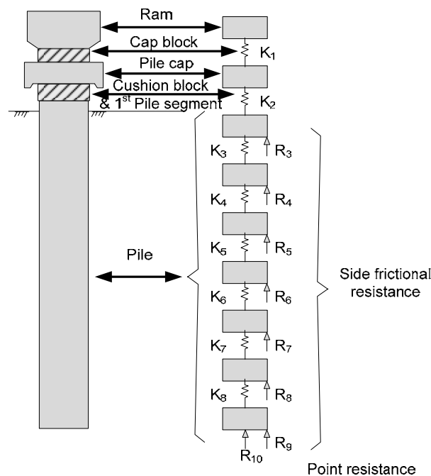
รูปที่ ค-3 ตัวอย่างแบบจำลองที่ใช้ในวิธีทฤษฎีคลื่นหน่วยแรงเชิงตัวเลข
